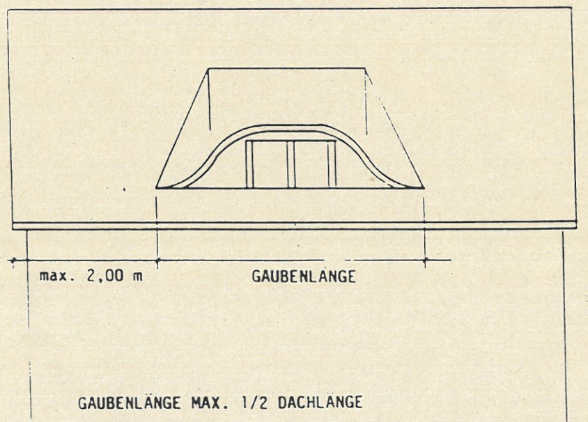
OCHSENAUGENGAUBE
